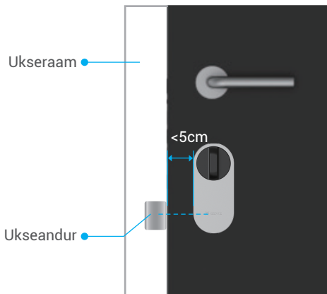
Eestvaade
